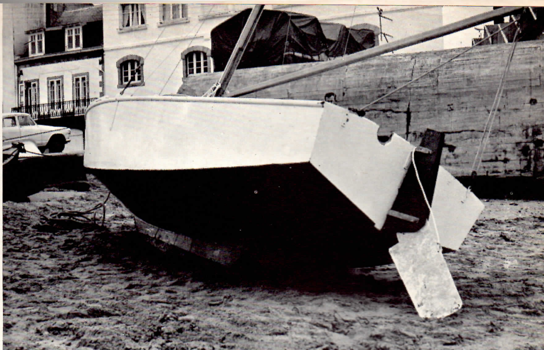
Le petit aileron porte-lest, placé sous la Cigogne, apporte une certaine stabilité, le rappel devenant moins important que sur la Caravelle.
